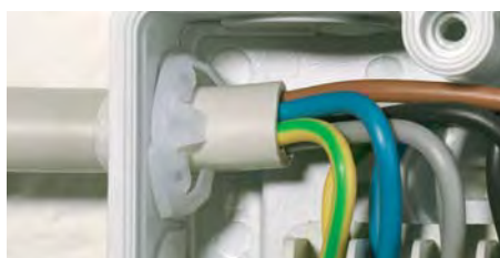
Фиксация кабеля с помощью фиксаторов KHN
