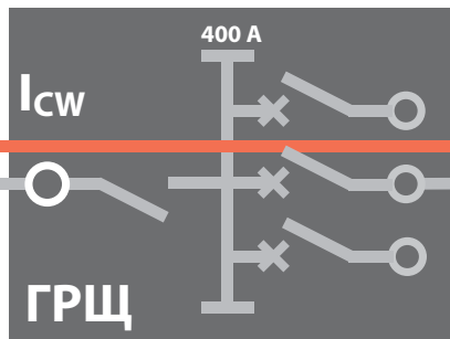
Главный распределительный щит (ГРЩ)
