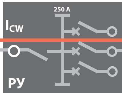
Распределительное устройство (РУ)
