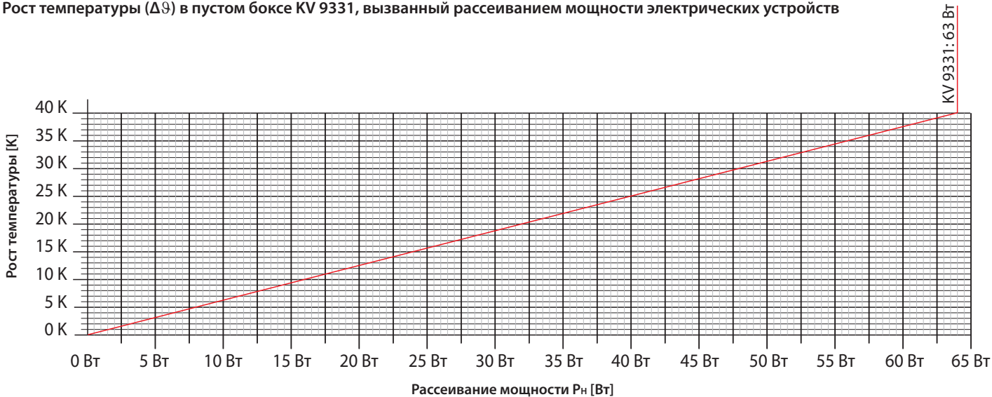
Рост температуры (Δθ) в пустом боксе KV 9331, вызванный рассеиванием мощности электрических устройств
