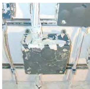
Ответвительная коробка с подключенными кабелями после испытаний..
