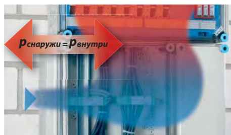
Вентиляционная заглушка
